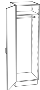
KS Klädskåp Djup 600 mm En flyttbar hylla, klädstång
