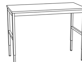
W100 Arbetsbord med undersarg och statvigavel ställbar. Bredd från 600 mm. Djup 600 eller 700 mm.
