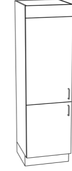
Högsåp för inbyggt kyl/frys HSK1-60 (hel lucka) HSK2-60 (delad lucka) Anpassas efter modell. Bredd 600 mm, Djup 600 mm, Höjd 1950 mm, 2100 mm.
