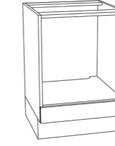
BSI60 Bänkskåp inb. ugn Anpassas efter modell. Bredd 600 mm, Djup 600 mm. Höjd 720 mm.
