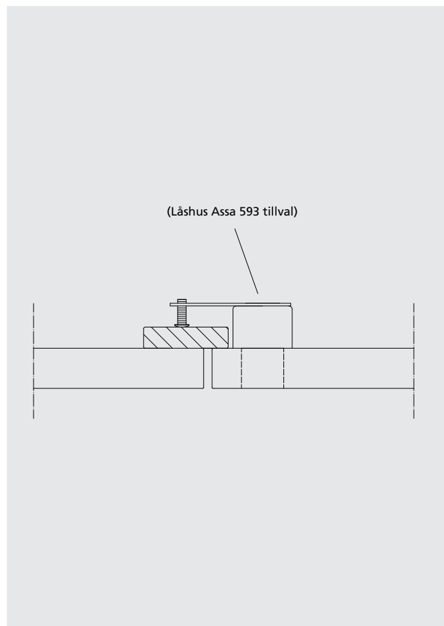
Pardörsmöte med anslagslist (vy från ovan)
