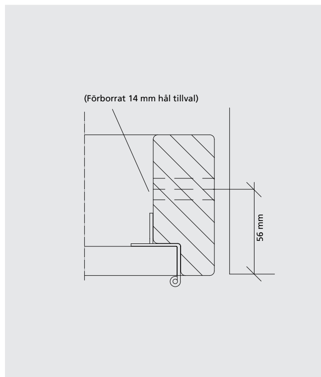
Karmsidostycke, gångjärnssida (vy från ovan)
