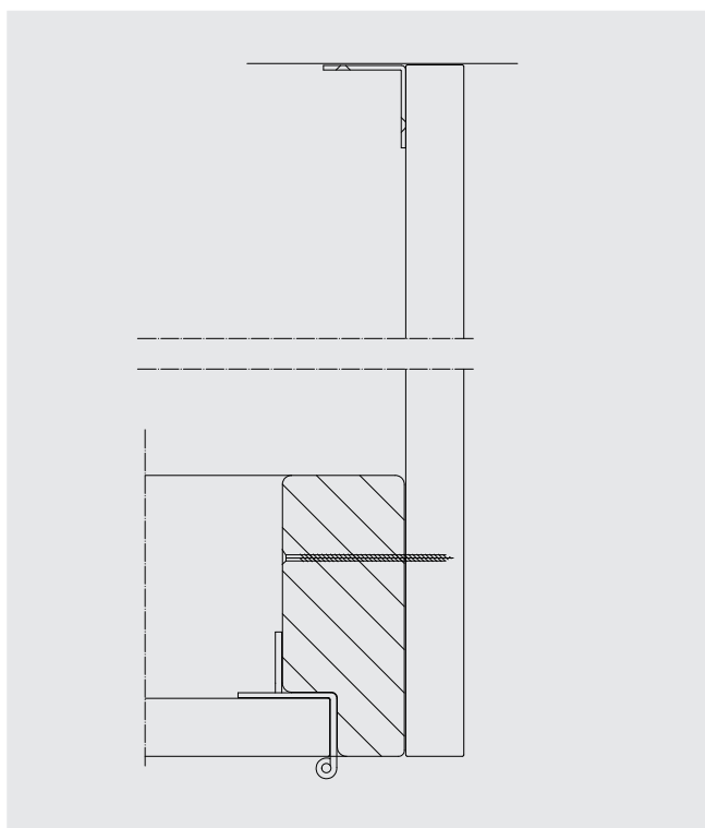
Utförande med sidoanslutning mot vägg – tillval (vy från ovan)
