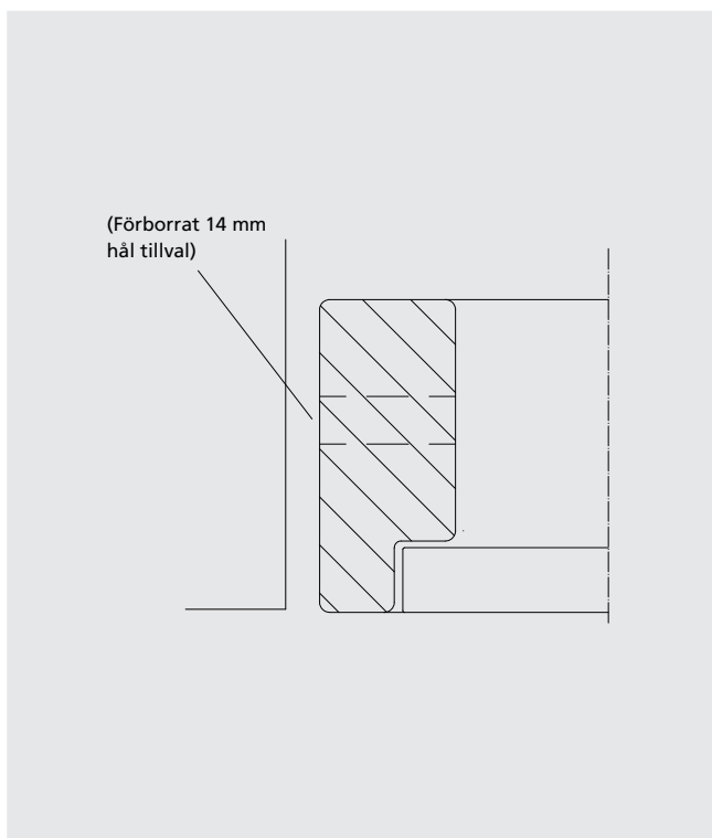
Karmsidostycke, anslagssida (vy från ovan)
