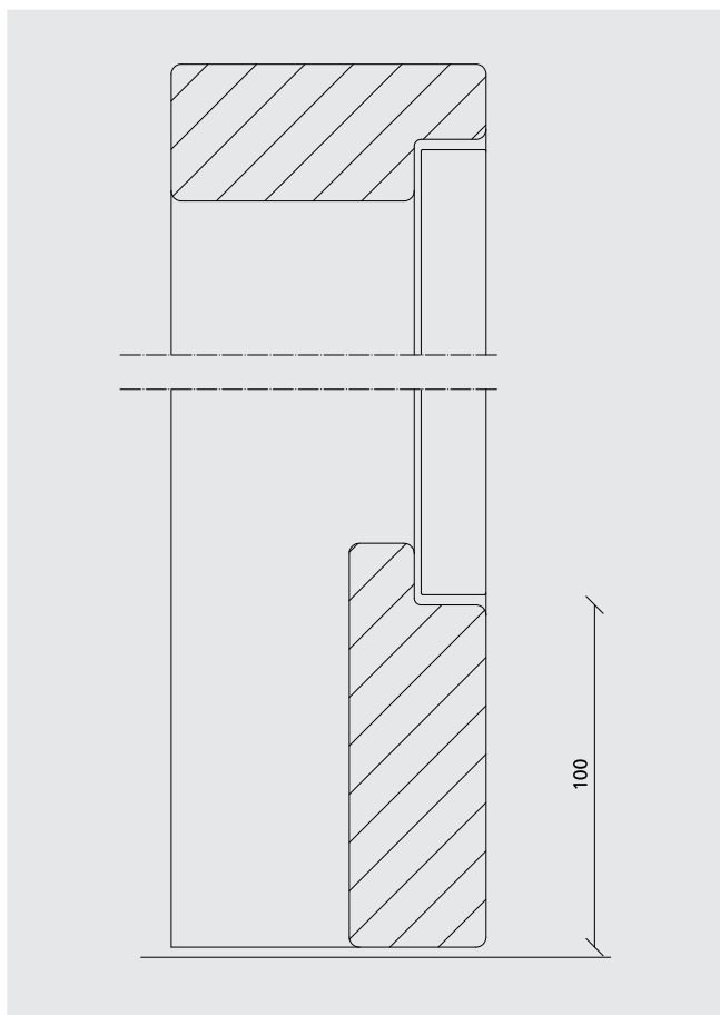
Förhöjd sockel, 100 mm – tillval (vy från sida)
