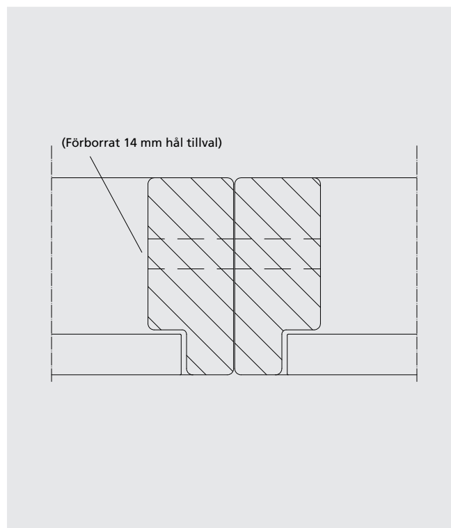
Anslutningsdetalj vid seriekopplade fronter (vy från ovan)
