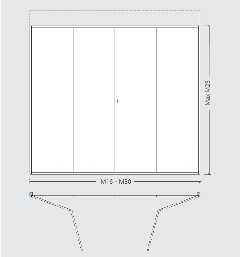
Fyrdelad lucka
