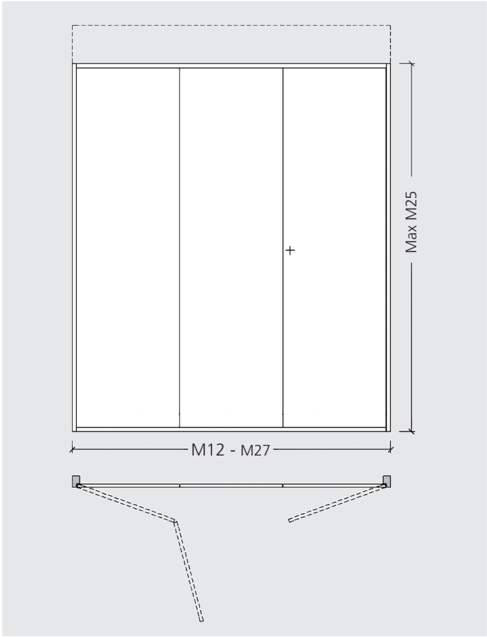
Tredelad lucka
