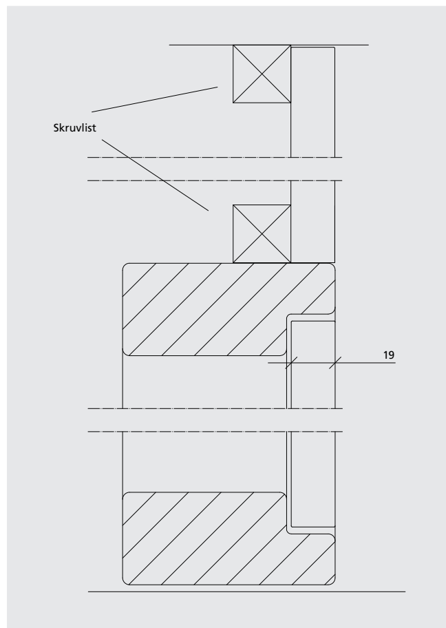
Utförande med takanslutning ovan karm – tillval
