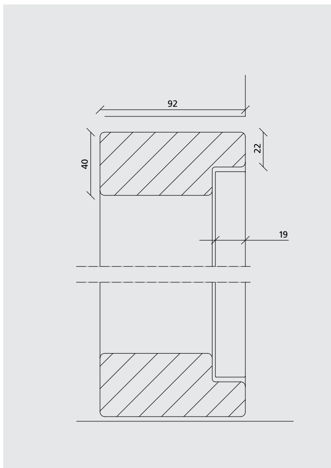
Karmprofiler uppe / nere (vy från sida)
