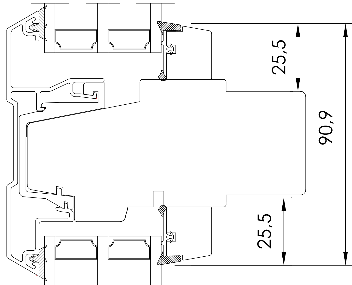
VERTIKALT SNITT TILLVAL - Flerluft Fasta delar med karmdelande tvärpost
