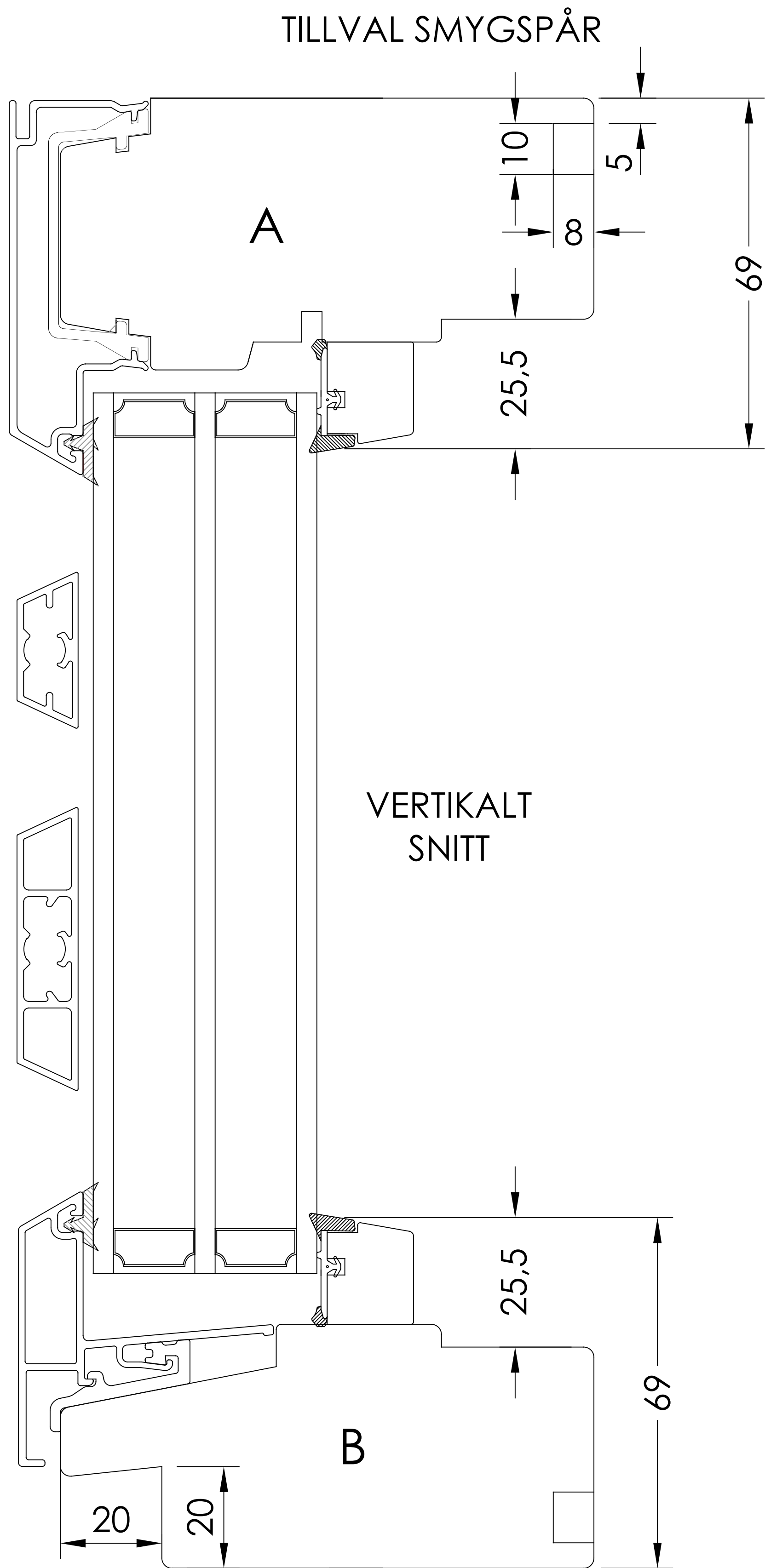
VERTIKALT SNITT TILLVAL - Norgenäsa
