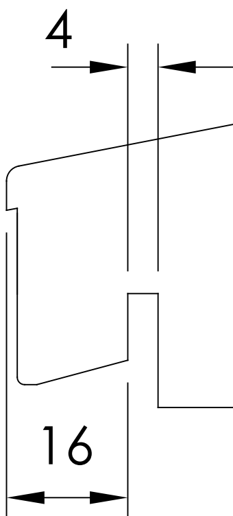
VERTIKALT SNITT TILLVAL - Norgenäsa
