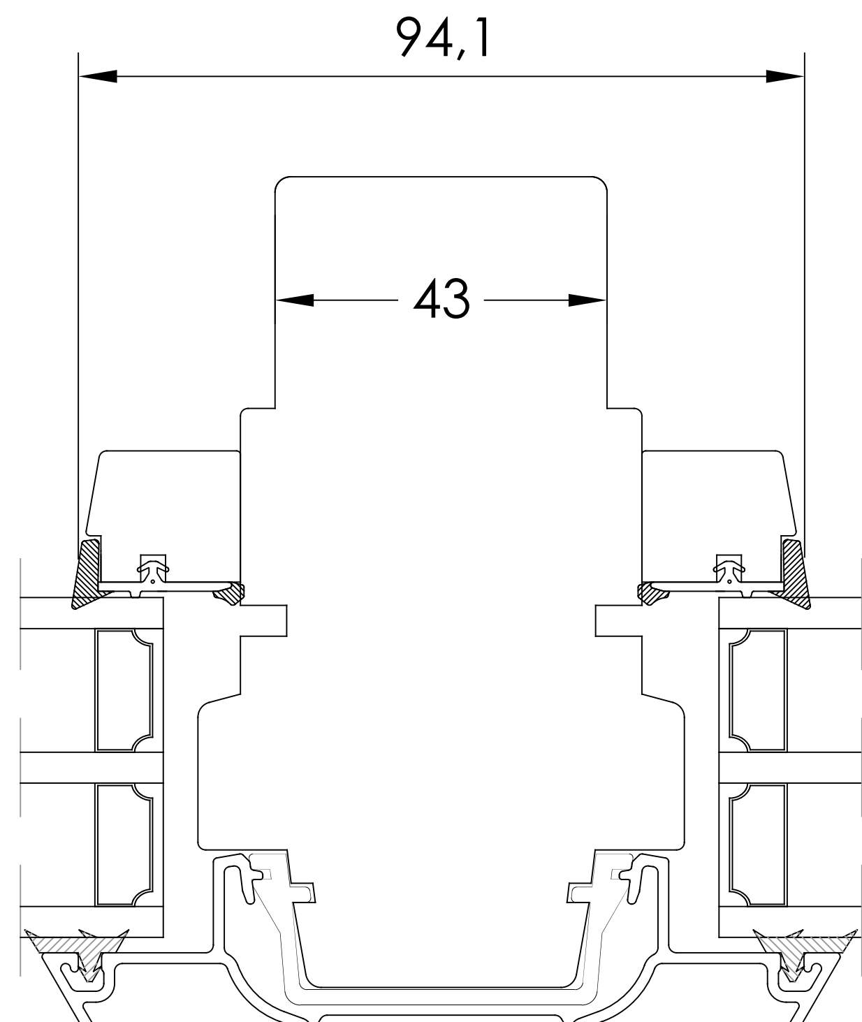
HORISONTALT SNITT TILLVAL - Flerluft Fasta delar med karmdelande post
