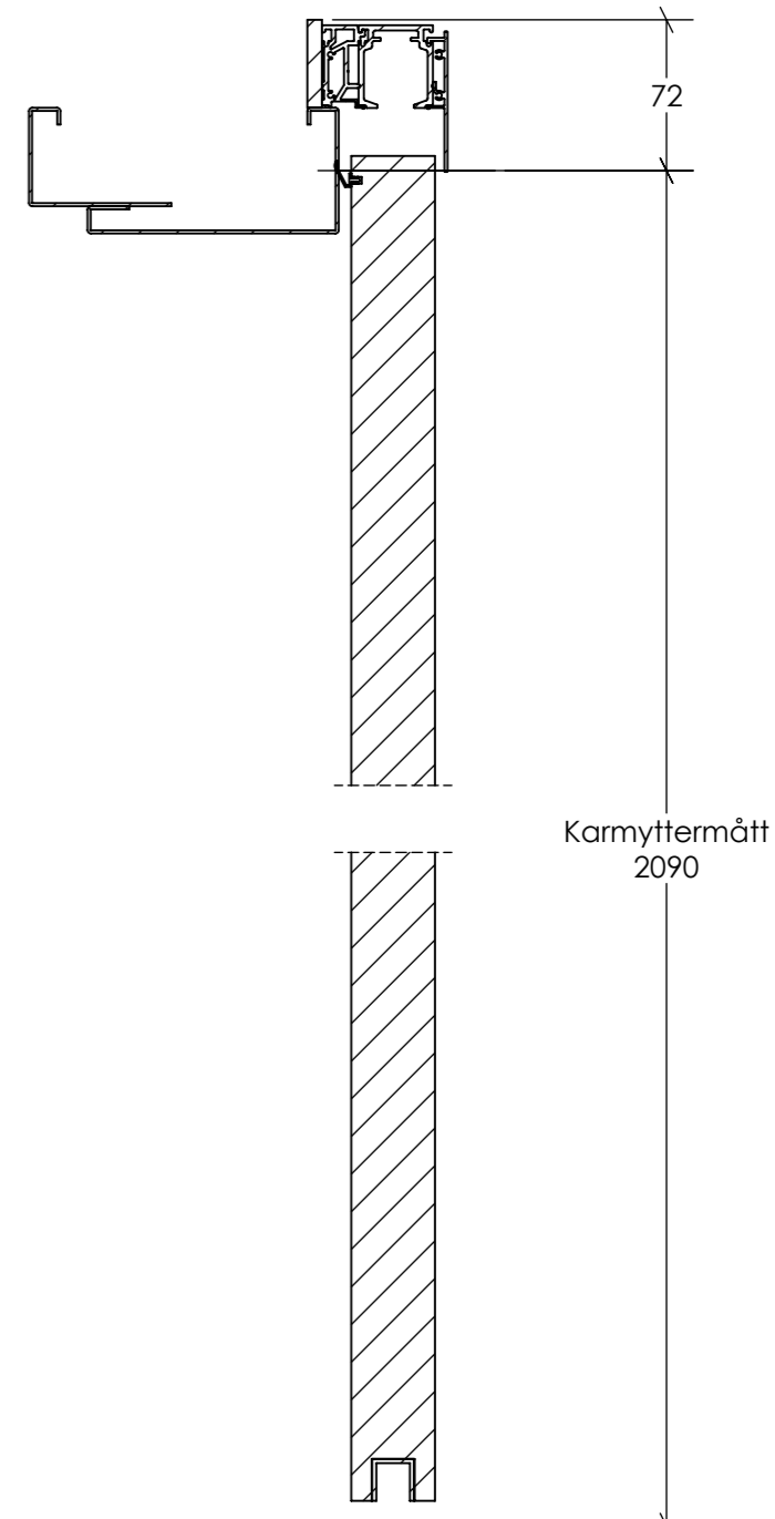
D-D 1 : 4
