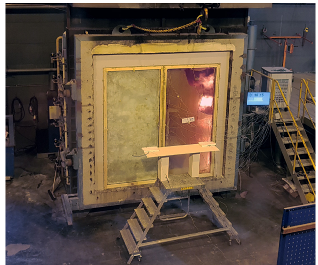
SSC Solid säkerhet under brandprovning.
